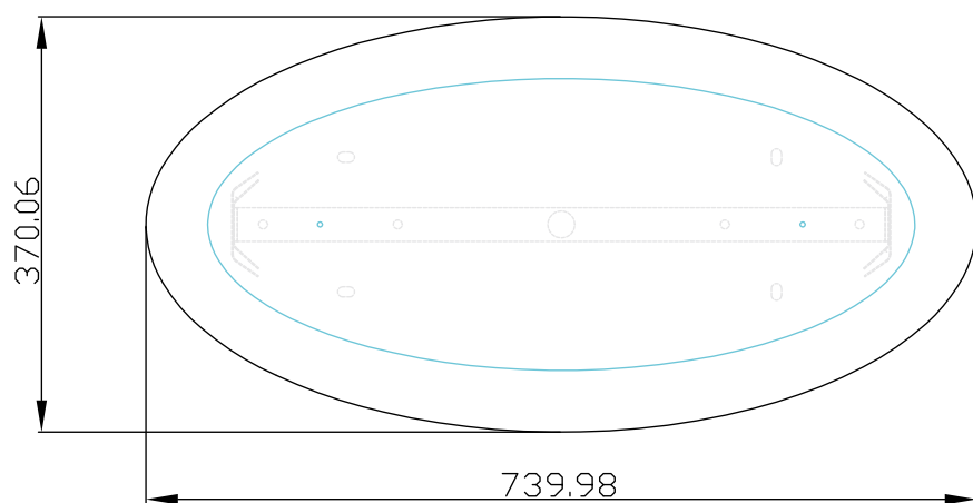
Telaio per espositore Totem 150 x 60
